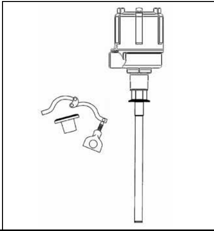
Sonda Sanitaria/3-A Protección Manga Delrin
