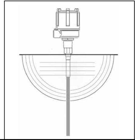
Sonda OEM Protección al Descubierto
