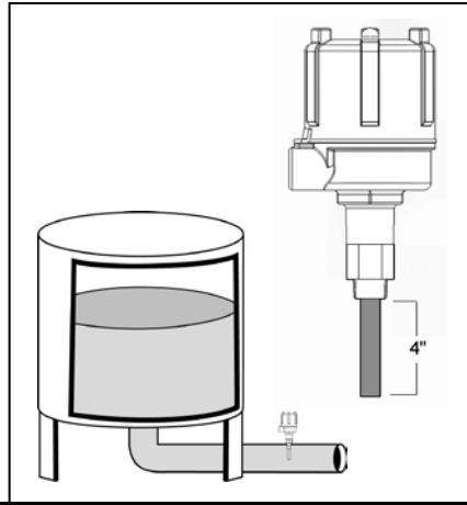
Sonda Cubierta con Delrin/Teflon Gruesa Sin Protección
